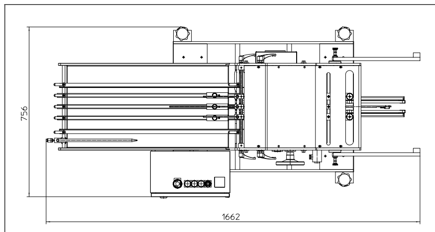
Abbildung 3: Grundriss
