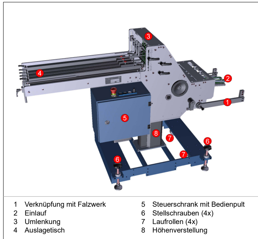
Abbildung 4: Stehendbogenauslage Typ XP-D 250.1
