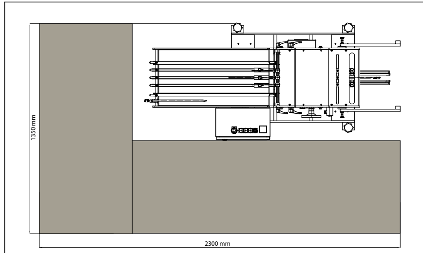
Abbildung 2: Arbeitsbereich
