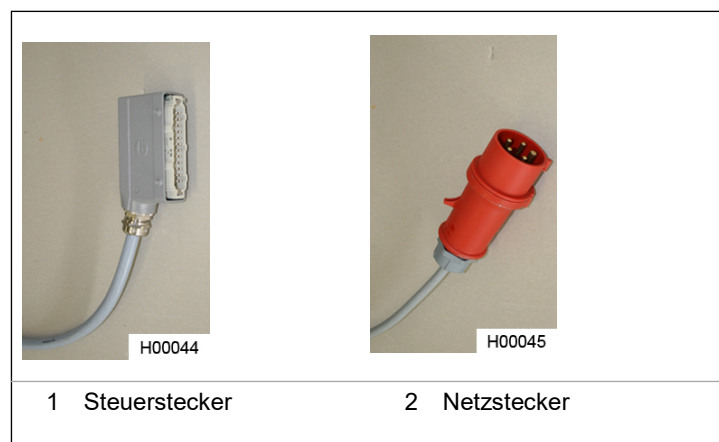
Abbildung 7: Anschlussstecker
