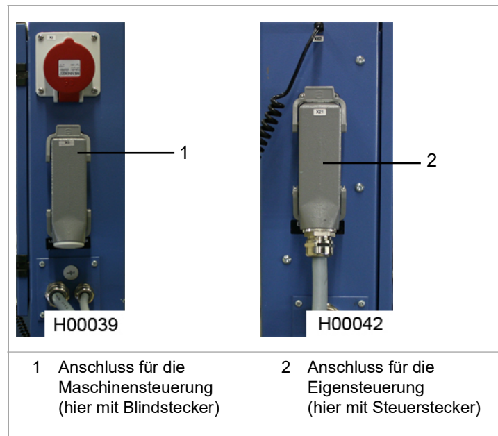
Abbildung 8: Anschlüsse für Eigensteuerung
