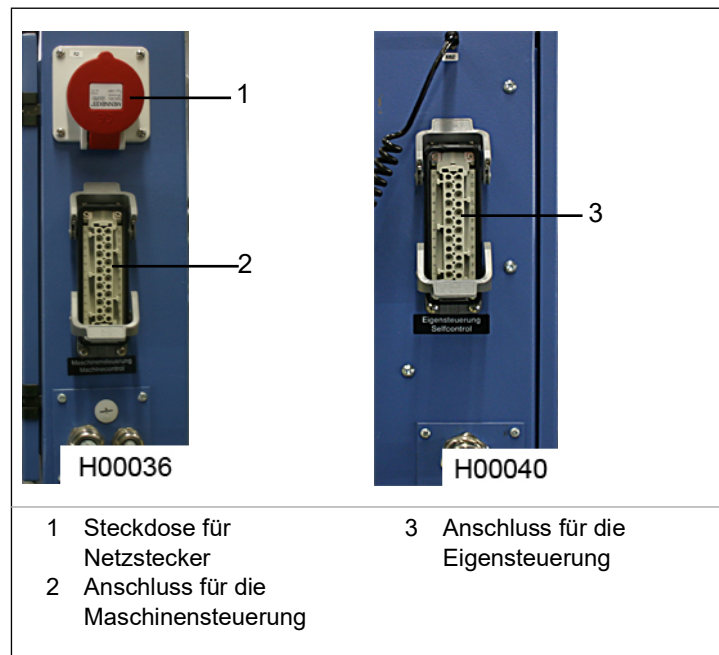
Abbildung 6: Netz- und Steueranschlüsse
