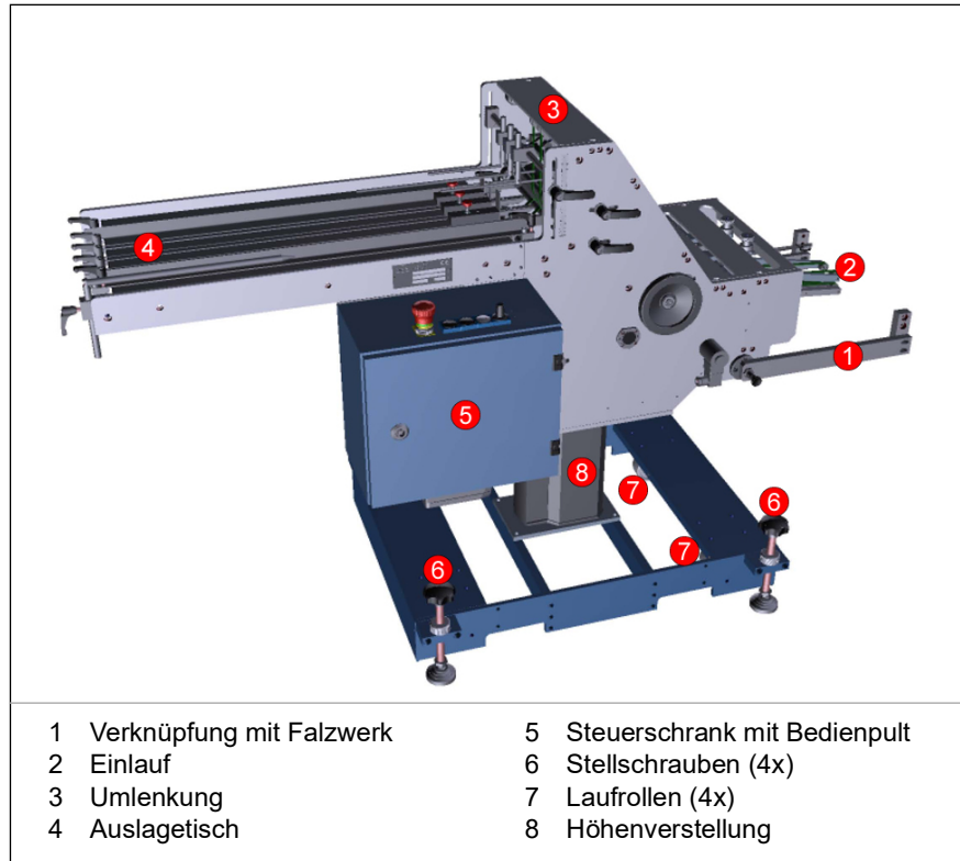
Abbildung 1: Stehendbogenauslage Typ XP-D 250.1
